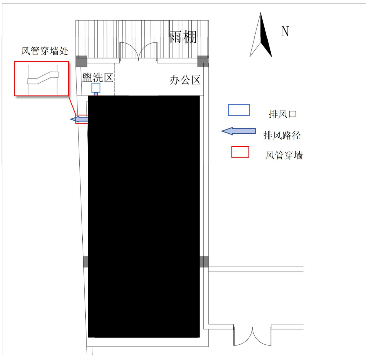
图 10-3 拟建放射性药品贮存仓库通风管道布置示意图
