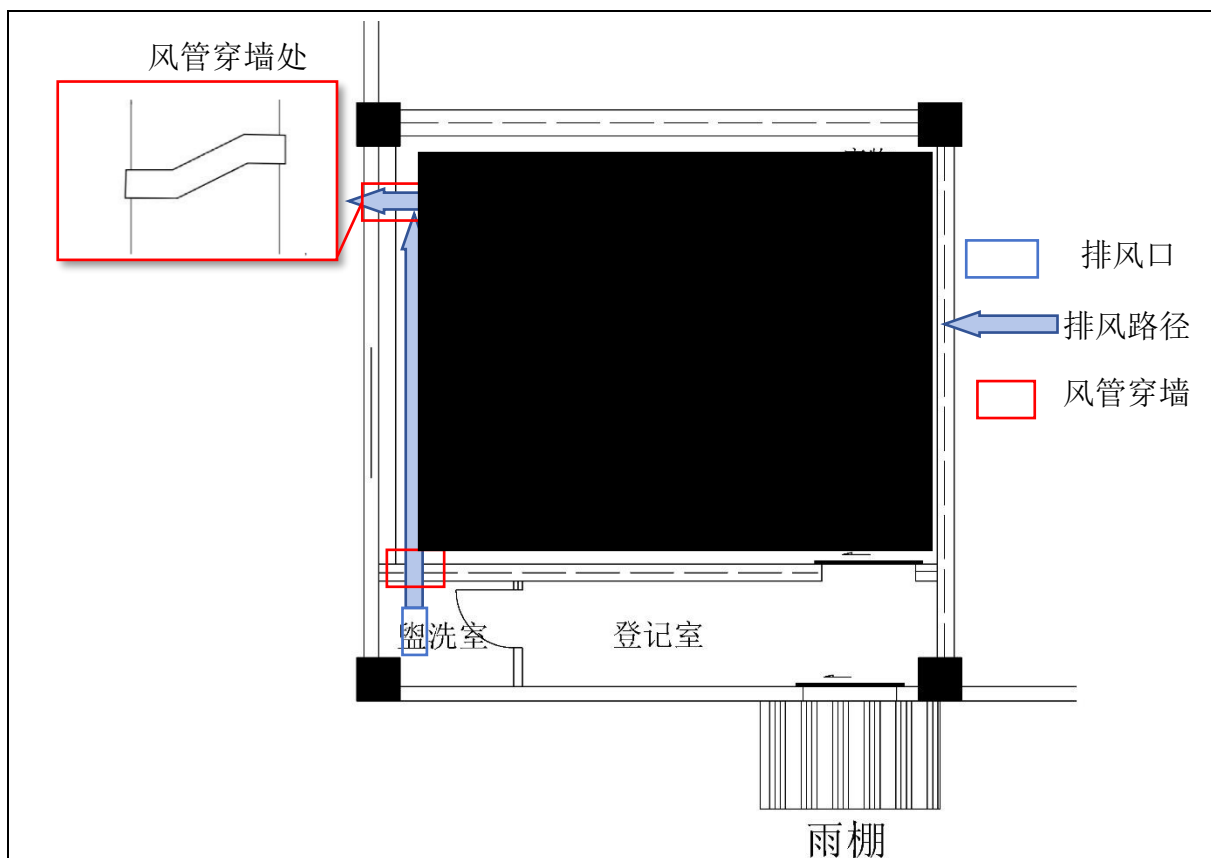
图 10-3 拟建放射性药品贮存仓库通风管道布置图
